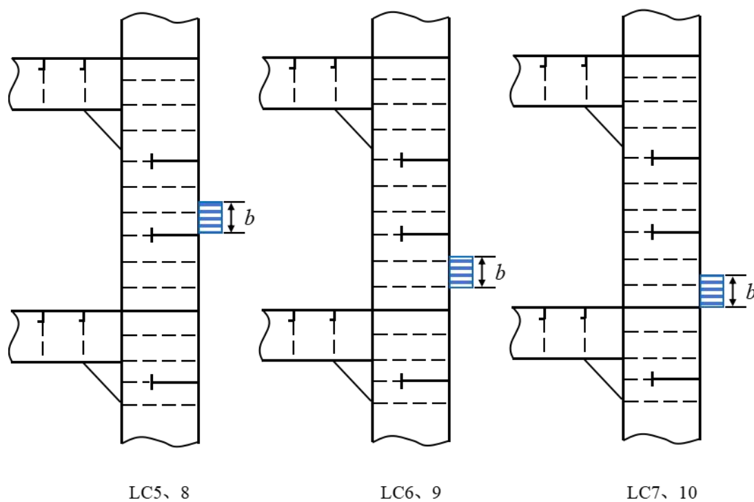
(d) Web frame/transverse diaphragm
