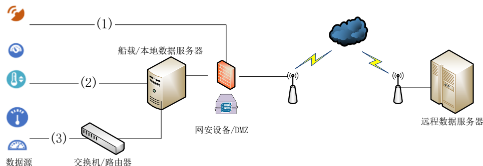
图 3.2.1.2 数据基础设施架构示例
