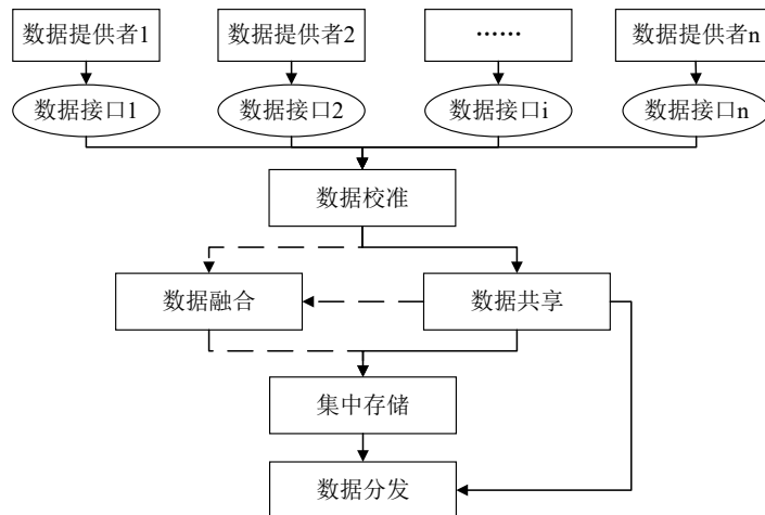
图 4.2.1.1 数据集成流程
