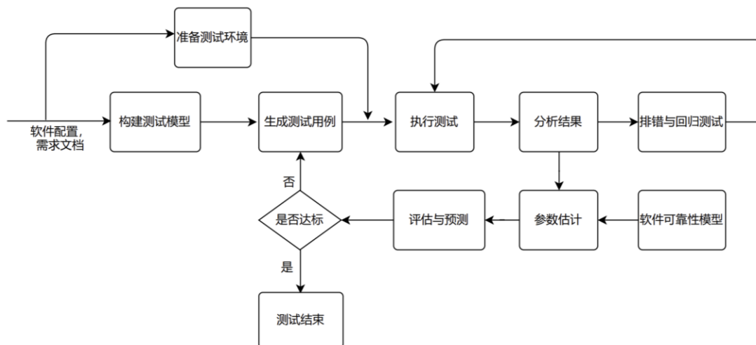
图 1.2.2.2 软件可靠性测试流程
