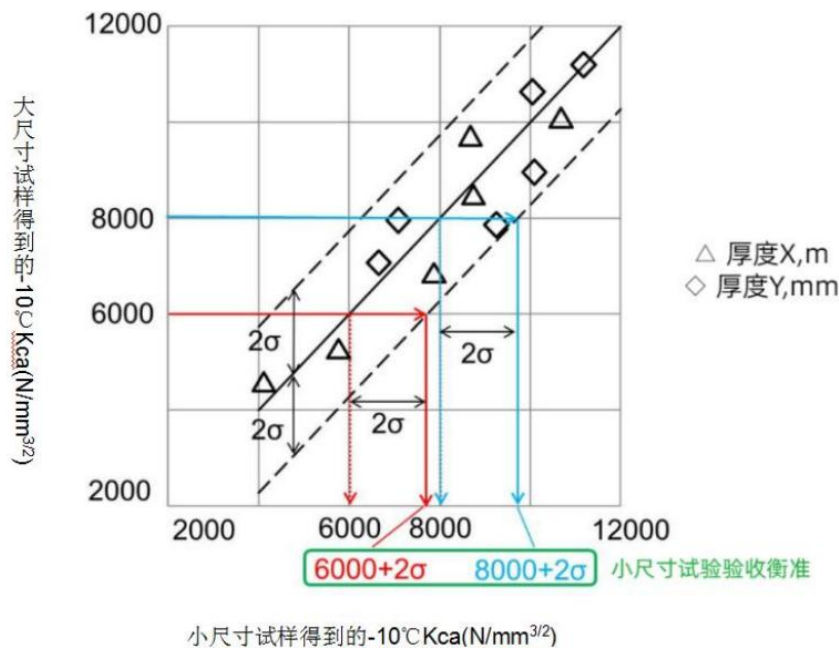
图 A5-2 通过脆性裂纹止裂韧性 ( K_{ca} ) 确定小尺寸试验验收衡准的示例
