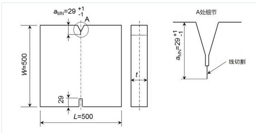
图 A4-1 冲击式试样的试样尺寸
