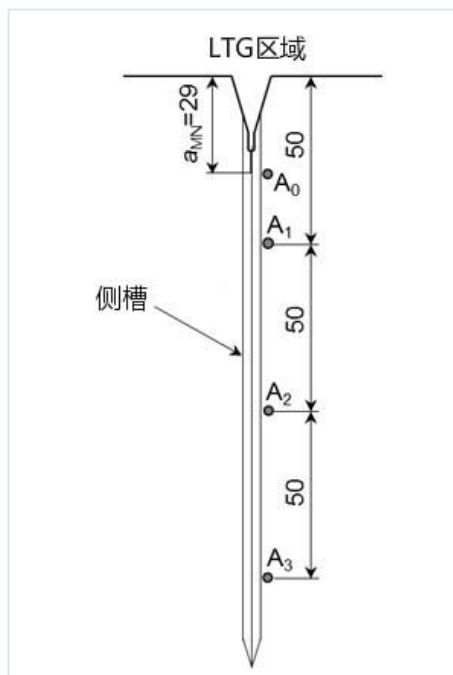
图 A4-5 LTG 区域和附加热电偶 A 0 详图
