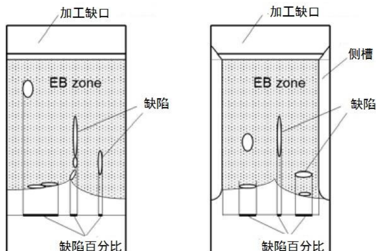
图 A4-8 缺陷百分比计算方法
