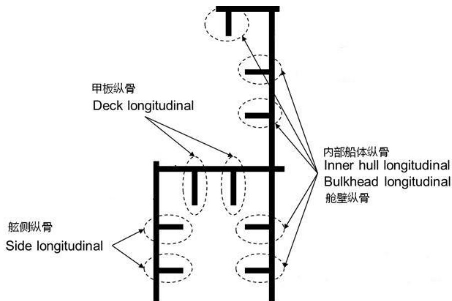
图 4.5.2 上部纵向构件
