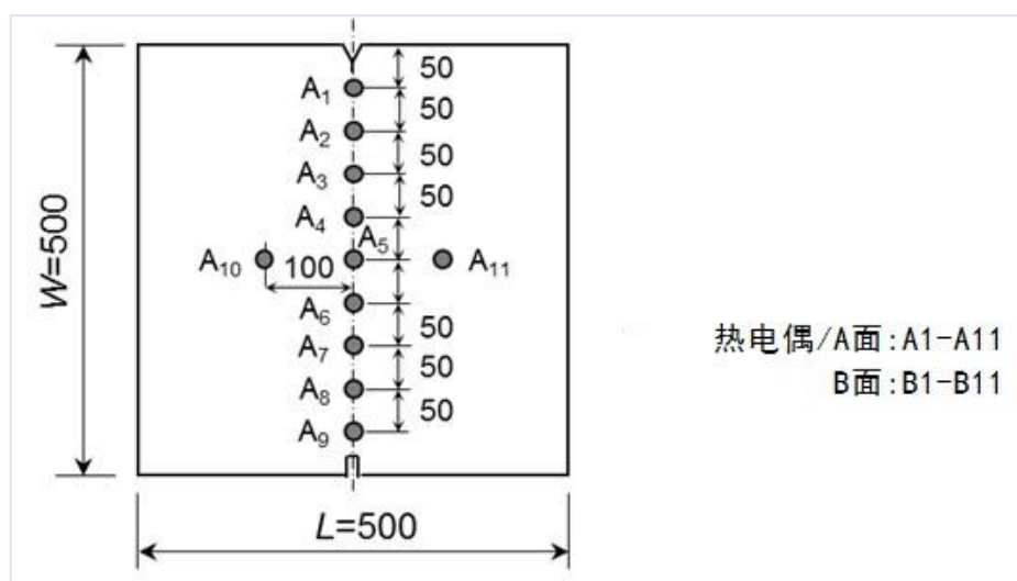
图 A4-4 温度测量位置
