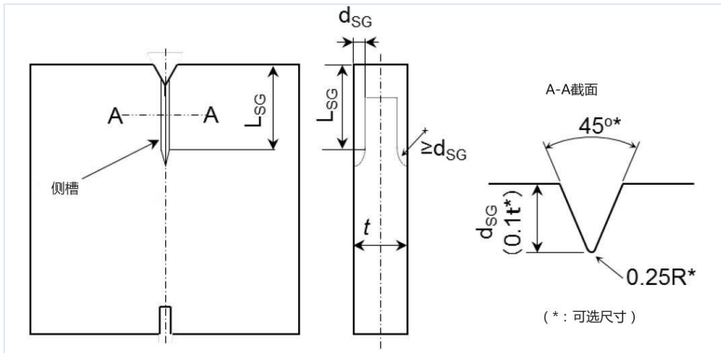
图 A4-2 侧槽形状和尺寸
