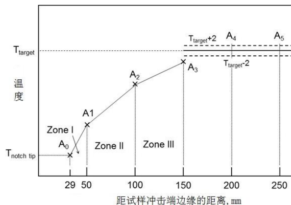
图 A4-6 LTG 区温度梯度剖面示意图
