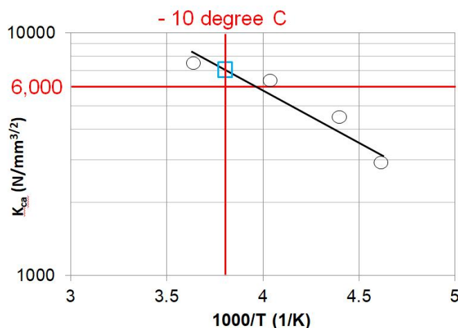
图 A3-1 评估 -10^\circ\text{C} 下 K_{ca} 的例子
