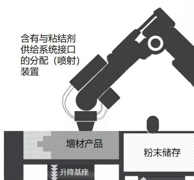
图 2.3.5 粘结剂喷射工艺
