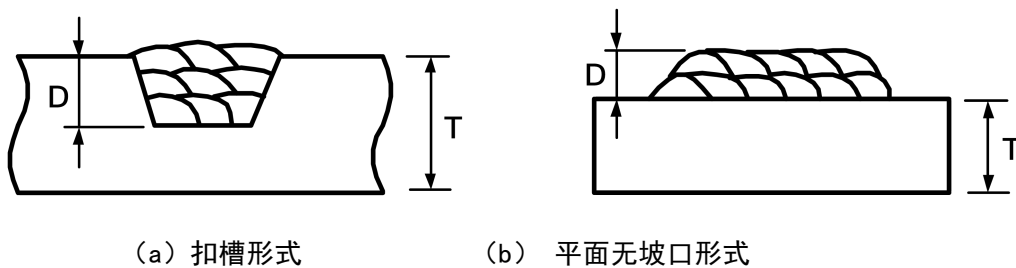
图 4.4.2-(2) 试件坡口形式
