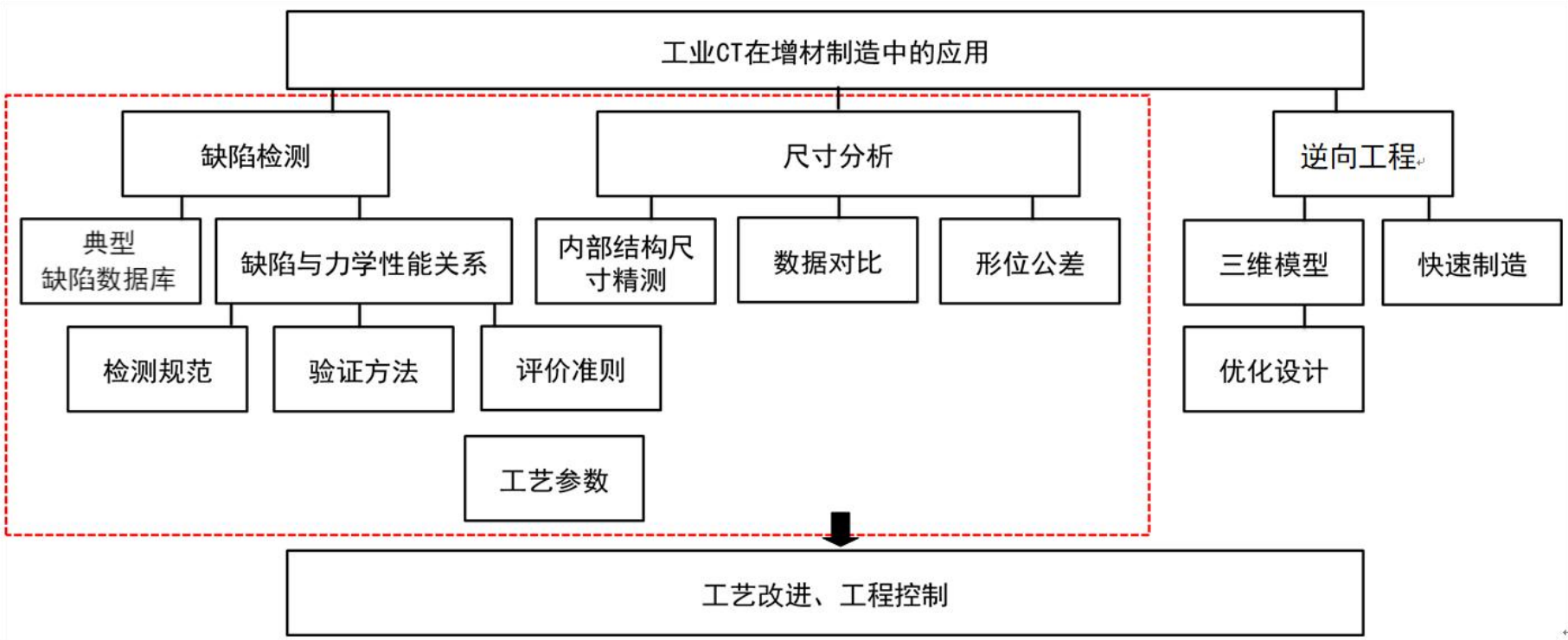
图 C.1 增材制造的工业 CT 检测应用流程图
