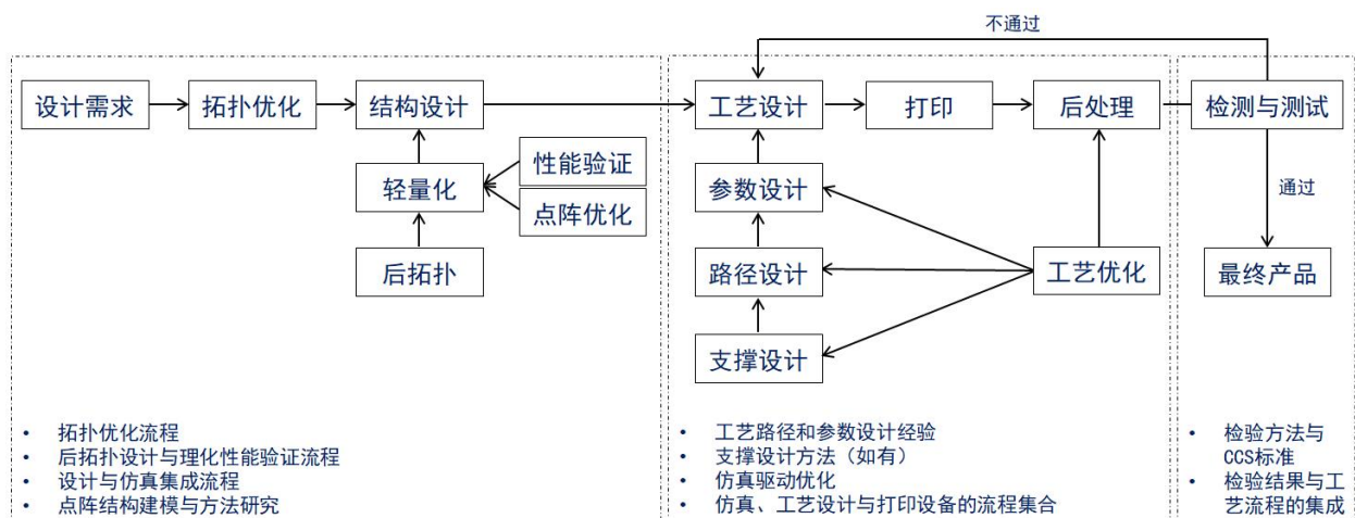
图 3.2.6 船舶与海工设施增材制造创新设计和制造一体化评估流程
