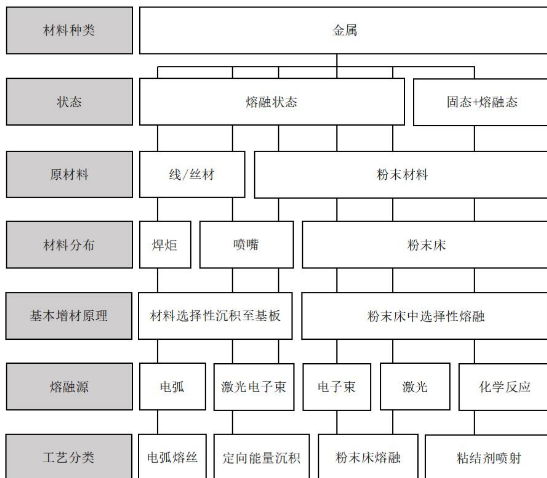
图 4.3.2.2 金属材料增材制造工艺流程图
