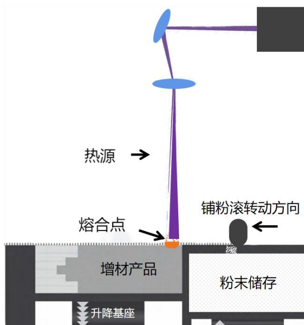
图 2.3.2 粉末床熔融工艺
