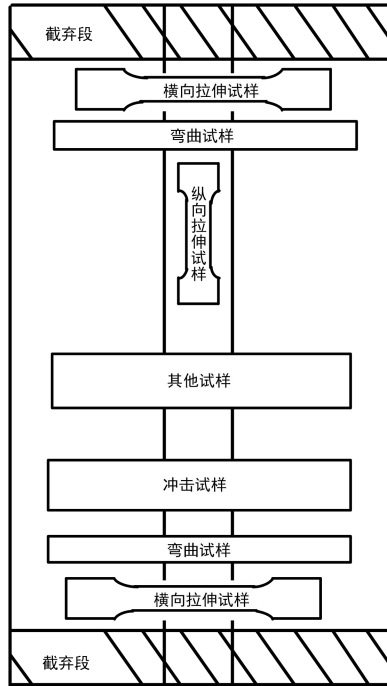
(a) 平板试件 ①②③
