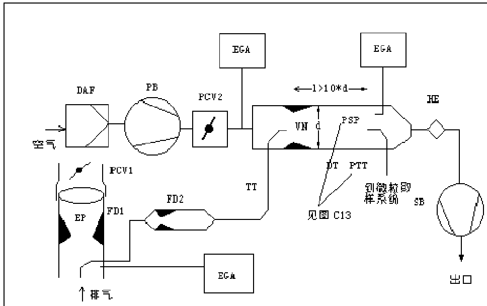
图 2.8 带双文丘里管或双流量孔，浓度测量，部分流取样的部分流稀释系统
