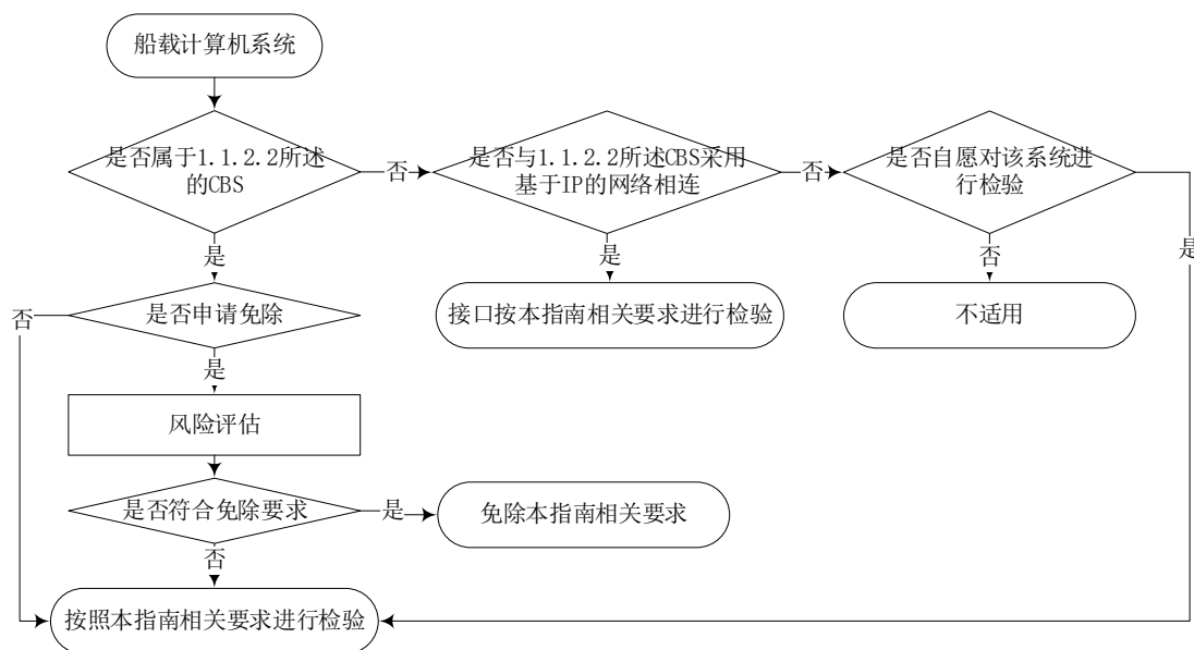
图 1.1.3.11 CBS 网络安全要求检验流程
