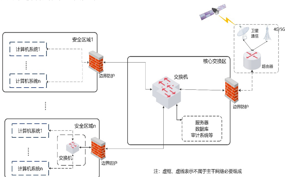
图 附录 3-1.1.1 船舶主干网络逻辑拓扑示意图
