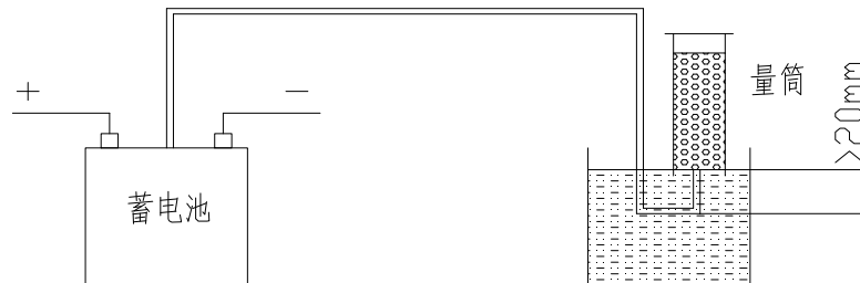
图 7.14 气体收集示意图
