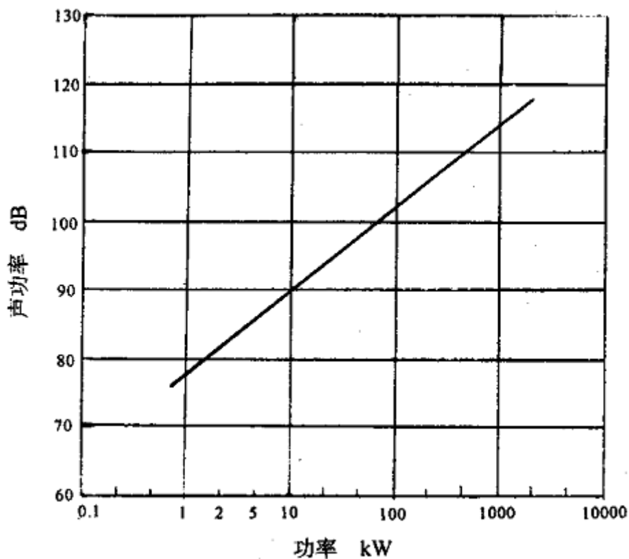
图 107.23.2(9) 噪声限值
