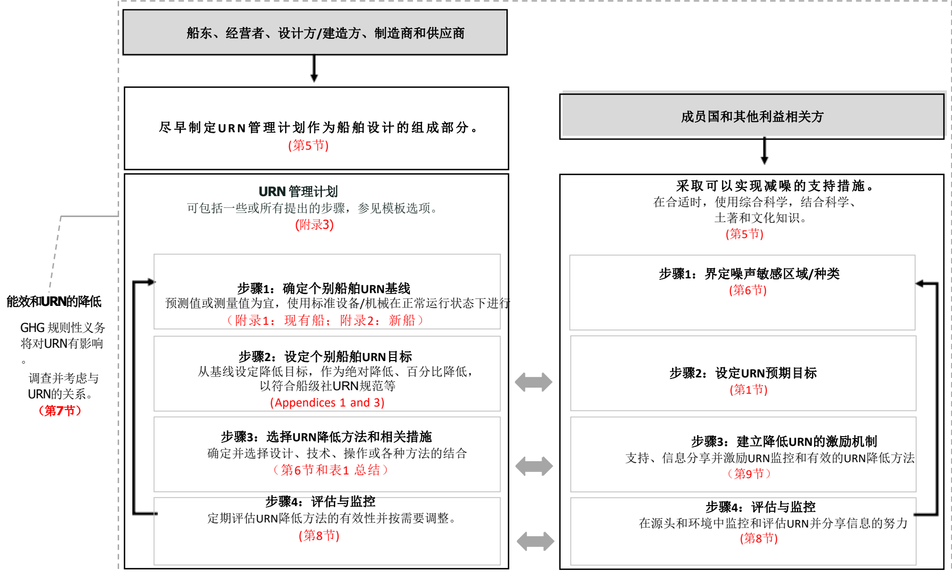
水下辐射噪声（URN）管理计划参考图
