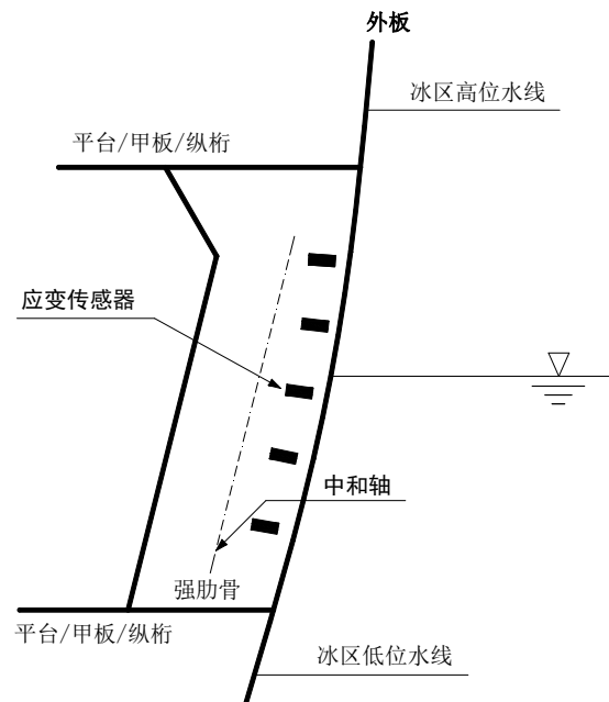
图 4.3.1 (2) 冰载荷反演强肋骨单向应变传感器布放示意图
