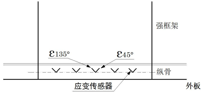
图 4.3.4 (1) 冰载荷反演纵骨双向应变传感器布放示意图
