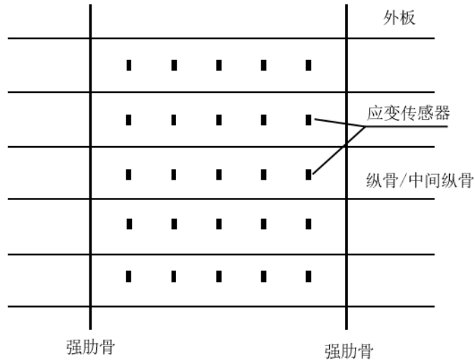
b. 纵骨架式
