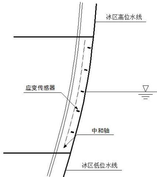
图 4.3.3 (2) 冰载荷反演肋骨单向应变传感器布放示意图
