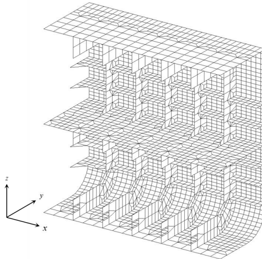
图 4.5.4 (2) 局部结构有限元模型
