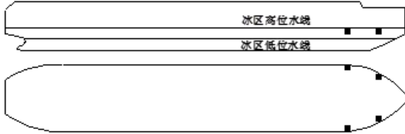
图 3.3.2(1) 监测传感器布放位置示意图
