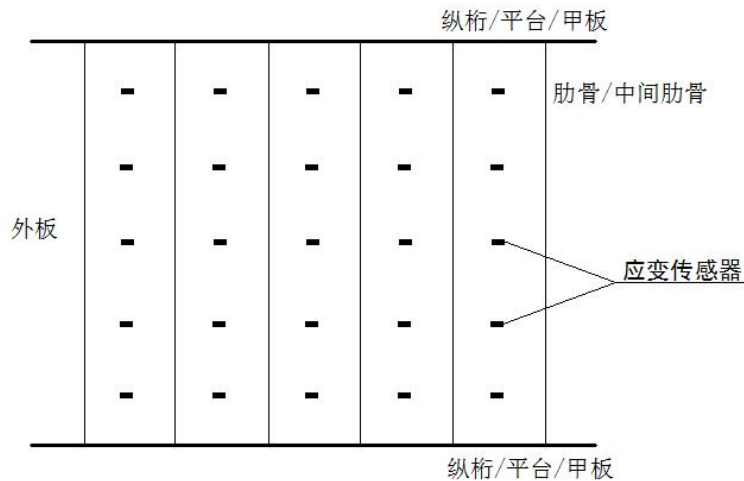
a. 横骨架式
