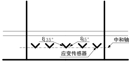
图 4.3.2 (1) 冰载荷反演纵桁双向应变传感器布放示意图
