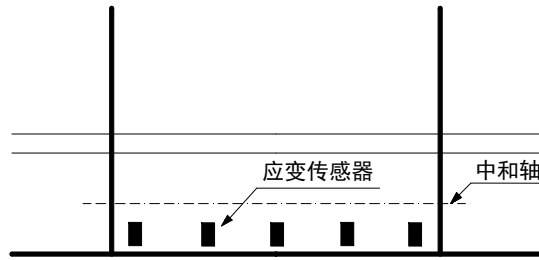
图 4.3.2 (2) 冰载荷反演纵桁单向应变传感器布放示意图
