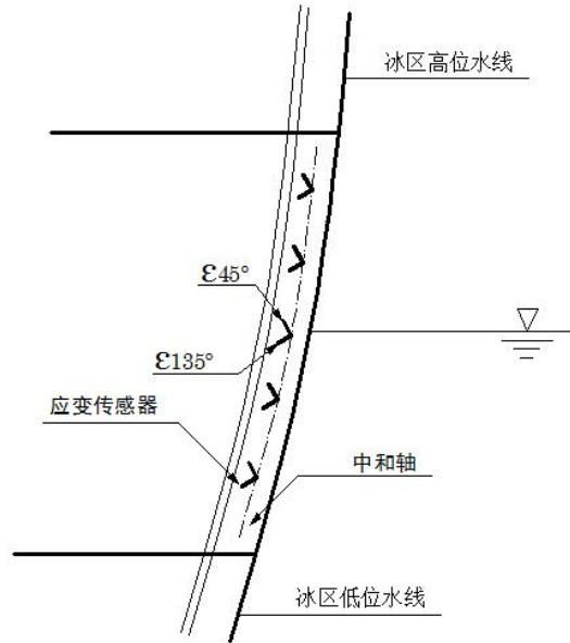
图 4.3.3 (1) 冰载荷反演肋骨双向应变传感器布放示意图
