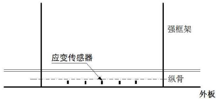
图 4.3.4 (2) 冰载荷反演纵骨单向应变传感器布放示意图
