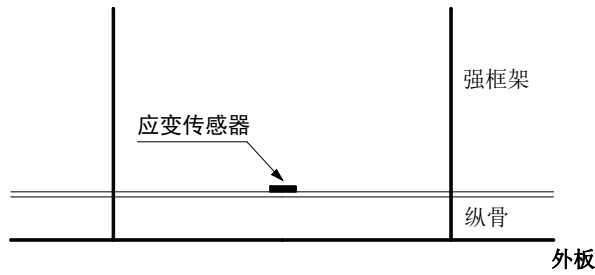
图 2.4.4 纵骨应变监测布放示意图
