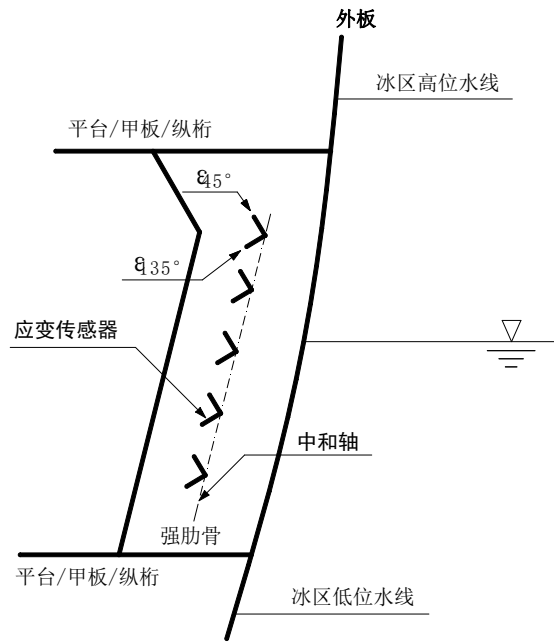
图 4.3.1 (1) 冰载荷反演强肋骨双向应变传感器布放示意图
