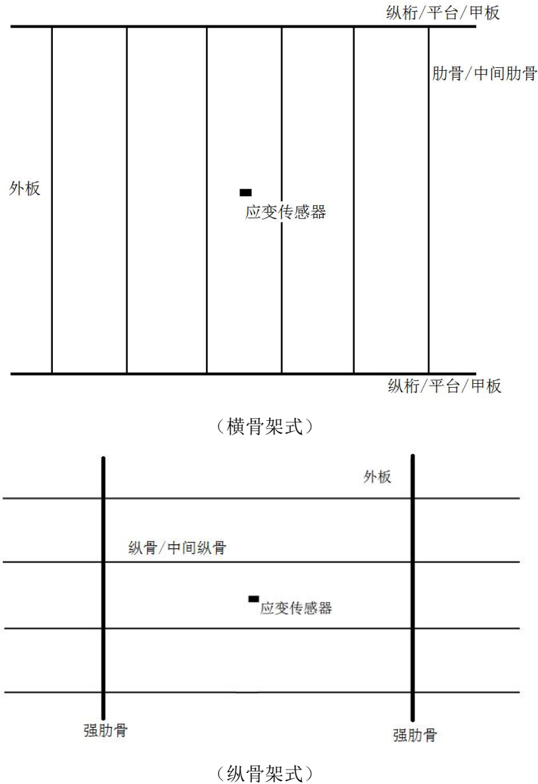
图 2.4.6 船体外板应变监测布放示意图
