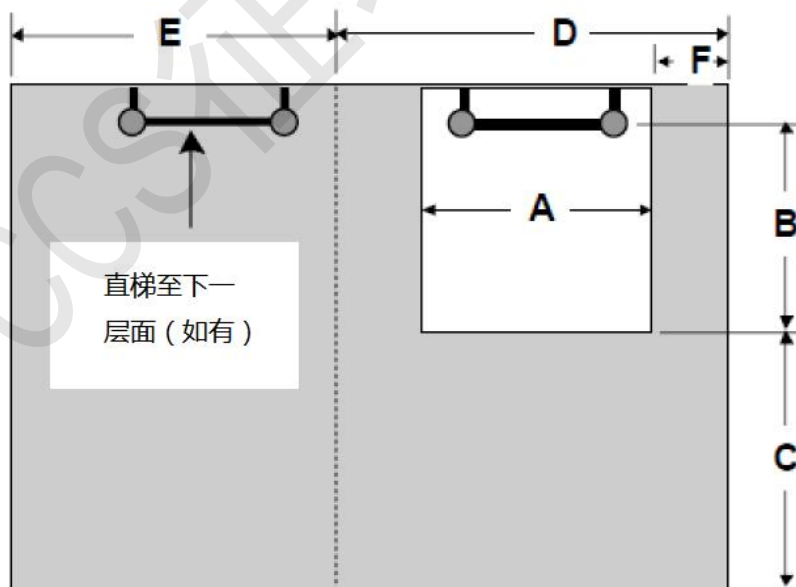
图 A. 1. 5. 5(4) 直梯至平台（直梯穿过平台）
