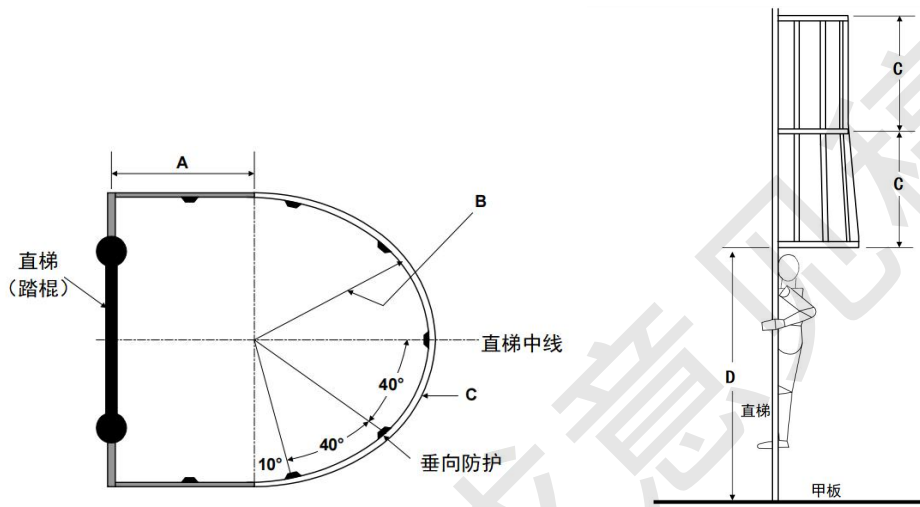
图 A. 1. 5. 5 (5) 直梯安全护笼
