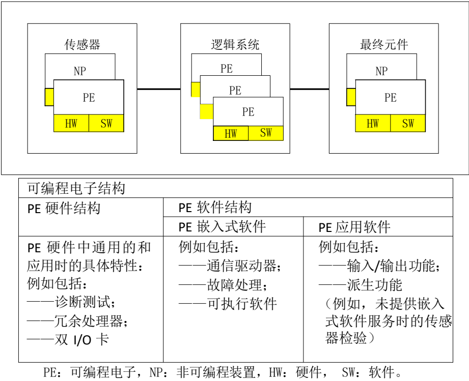
图附录 3-1.1.2 PE 硬件和软件结构的关系
