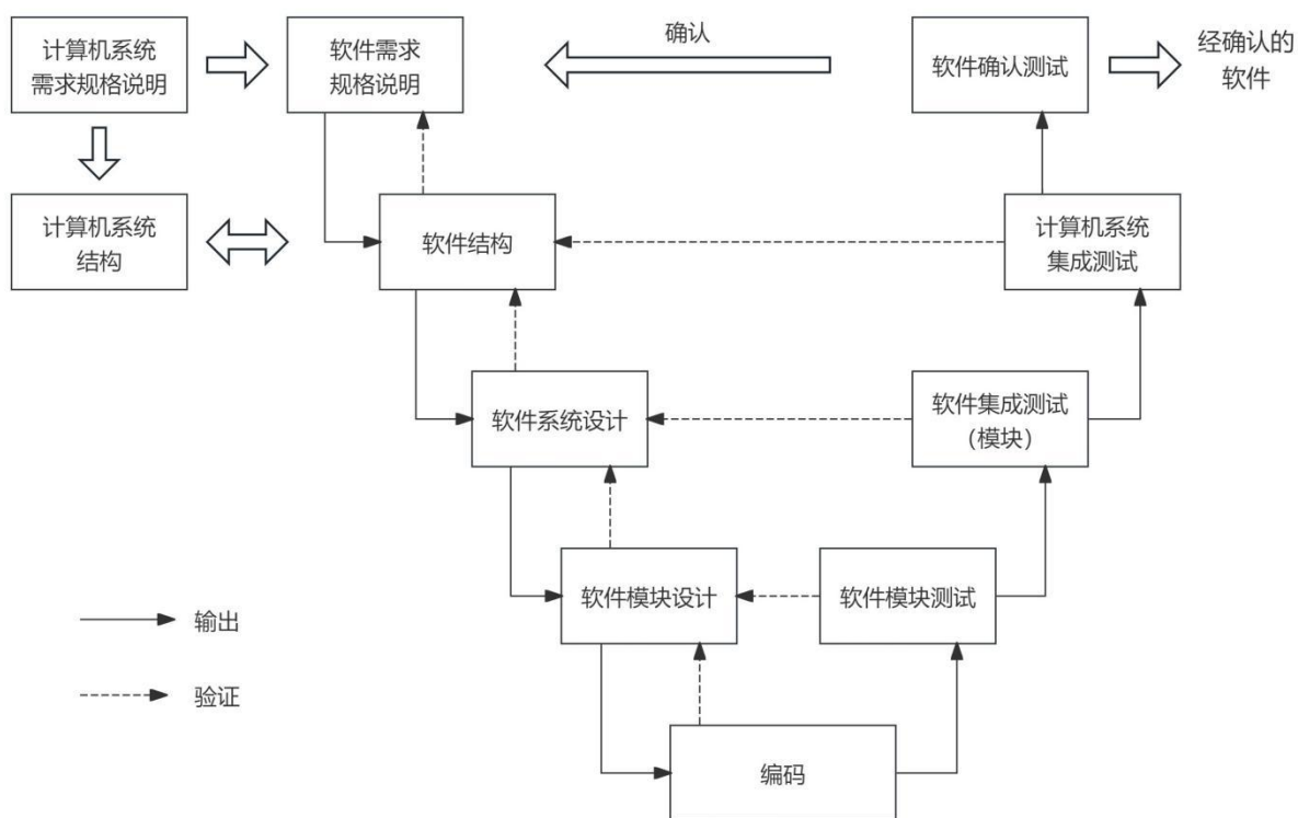
图 9.2.3-3 软件开发生命周期模型（V 模型）
