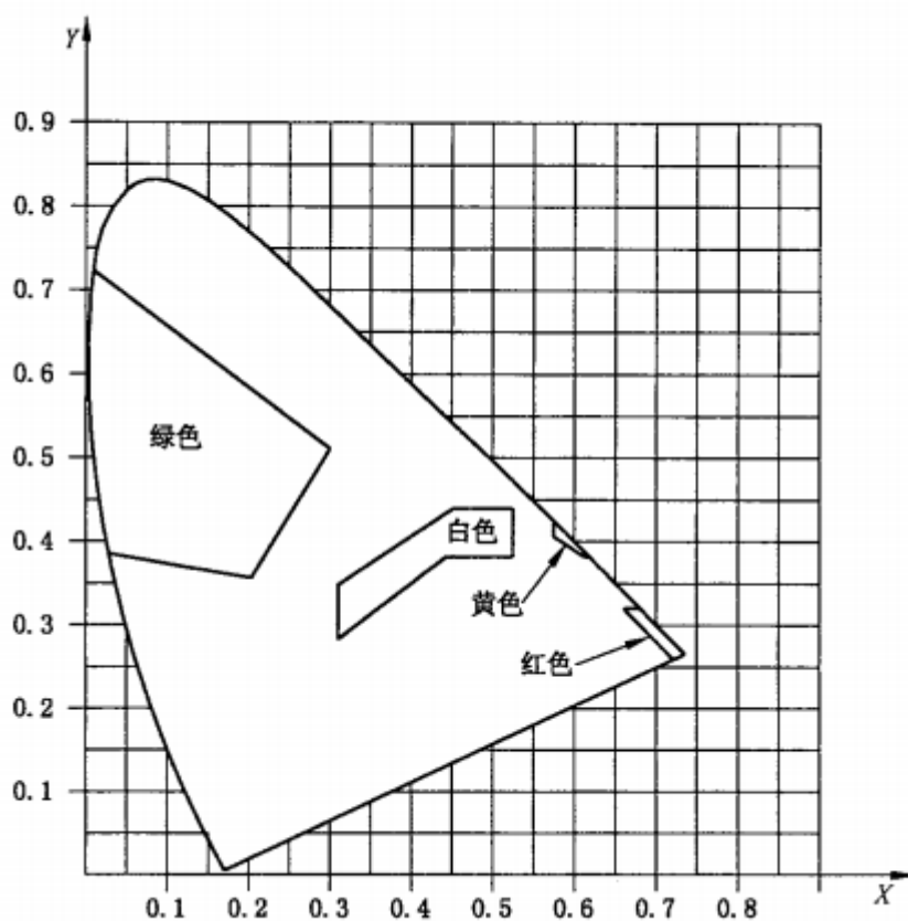
图 5.2.1 航行灯色度坐标
