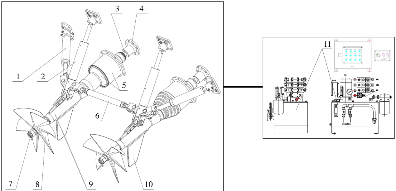
1 转舵油缸 2 纵倾油缸 3 输入轴 4 法兰联轴器 5 球座与球体 6 连杆 7 螺旋桨轴 8 螺旋桨 9 支架 10 舵板 11 液动力单元和控制箱方向控制装置
