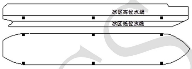
图 10.6.3.3 冰区加强船舶传感器布置示意图
