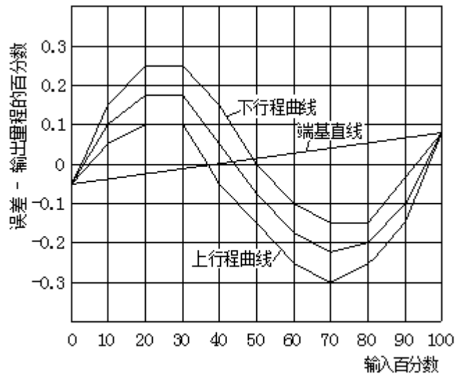
图 5.3.3(1) 偏差曲线
