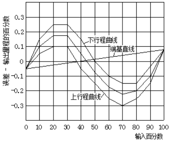
图 5.3.3(1) 偏差曲线
