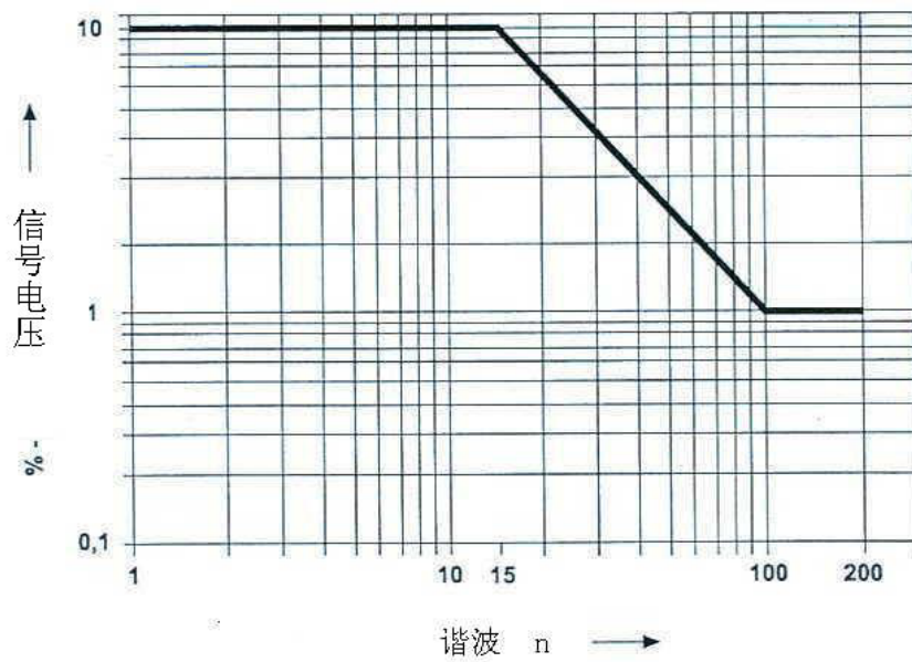
图3.8.2 交流供电设备低频传导抗扰度试验的信号电压
