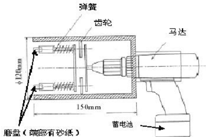
图 1 取样设备示意图
