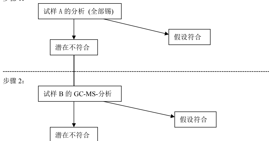
图 B 有机锡化合物二个步骤分析程序的流程图
