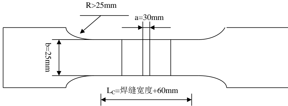
图 9(2) 拉伸试样图
