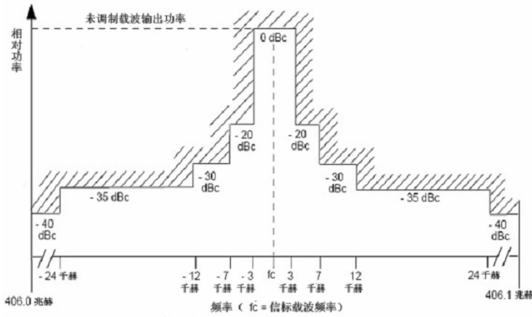
图 5.2.12 460.0MHz~406.1MHz 频带内的杂散发射分布图
