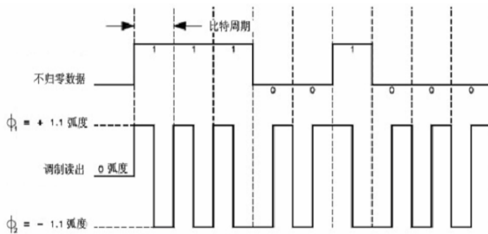
图 5.2.13 数据编码和调制示意图
