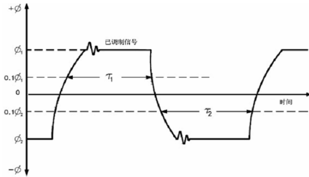
图 5.2.14 (2) 调制对称性的定义
