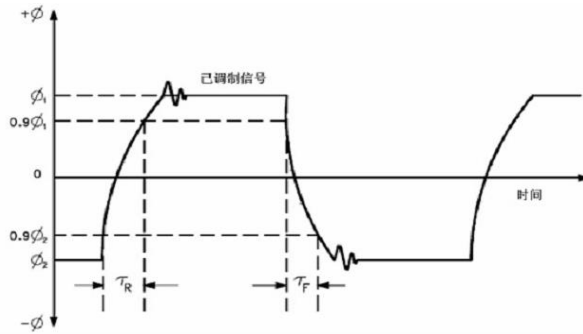
图 5.2.14 (1) 调制上升和下降时间的定义
