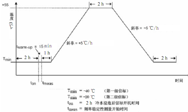
图 5.2.18 温度梯度
