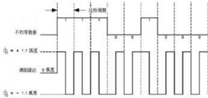
图 5.2.13 数据编码和调制示意图
