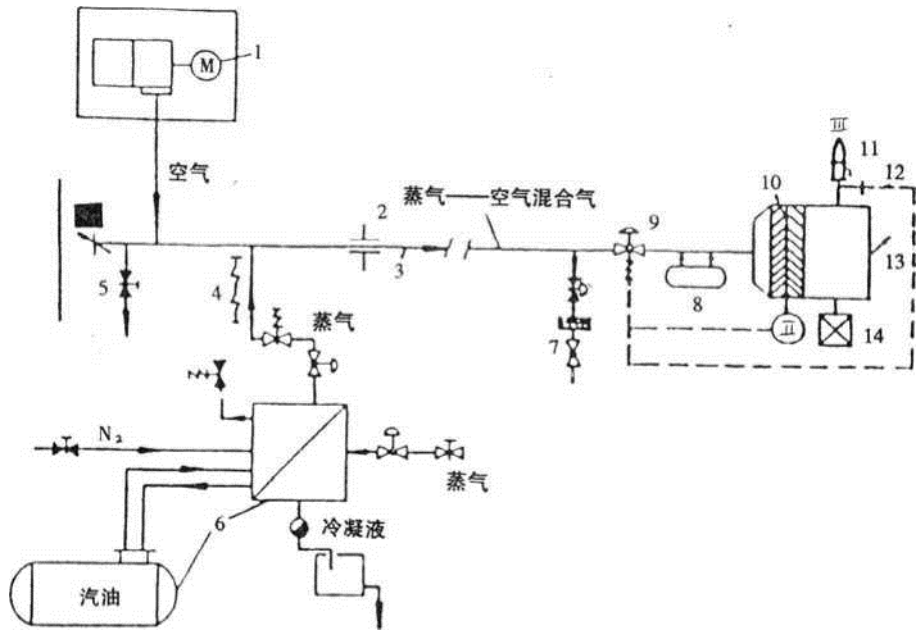
1. 变速风机；2. 容积流量计；3. 管子（直径 50mm，长约 30m）；4. 热蒸气管；5. 空气旁通阀；6. 蒸发器和液体贮存柜；7. 蒸气/空气—混合气旁通装置；8. 灭火剂；9. 控制与速闭阀；10. 保证试验装置安全；带有温度控制的防爆波形带；11 被试验的高速阀；12. 火焰探测器；13. 爆破膜片；14. 深度指示器；15. 气柜
