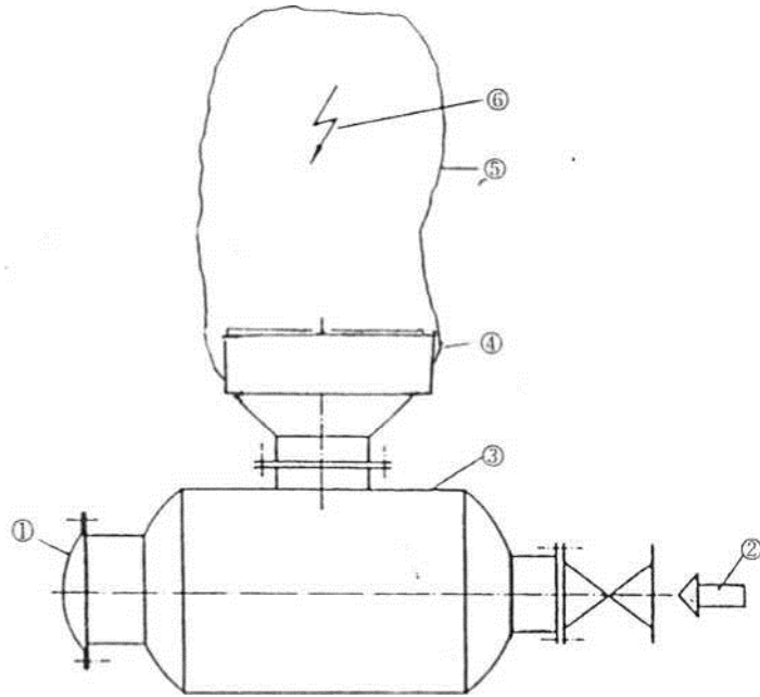
1. 爆破膜片（塑料）；2. 爆炸混合气入口；3. 气柜；4. 阻焰装置；5. 塑料袋；6. 点火源
