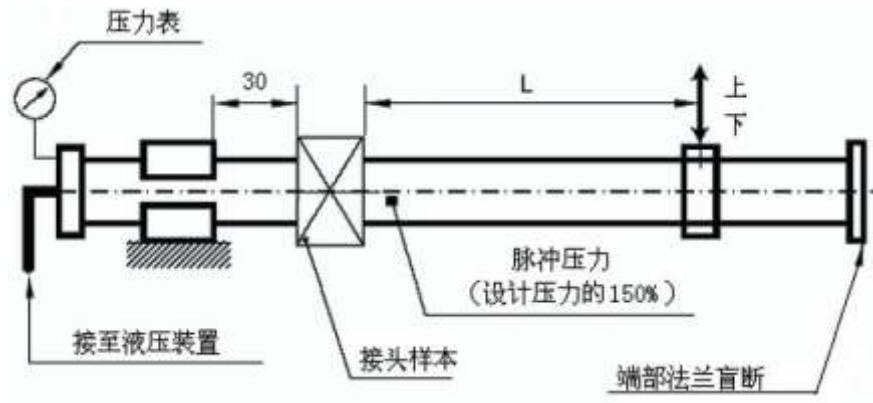
图7.6.2(1) 振动(疲劳)试验装置示意图
