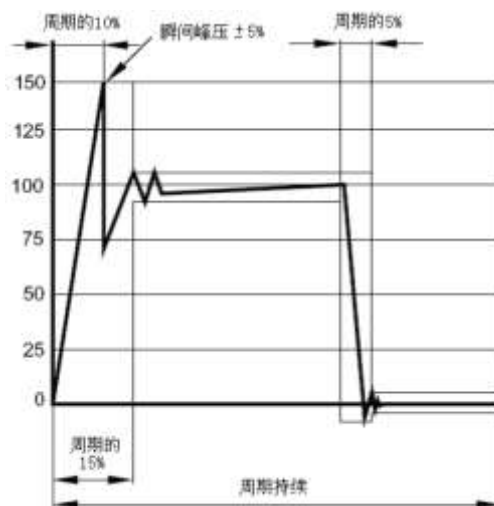
图7.6.3 压力脉冲图
