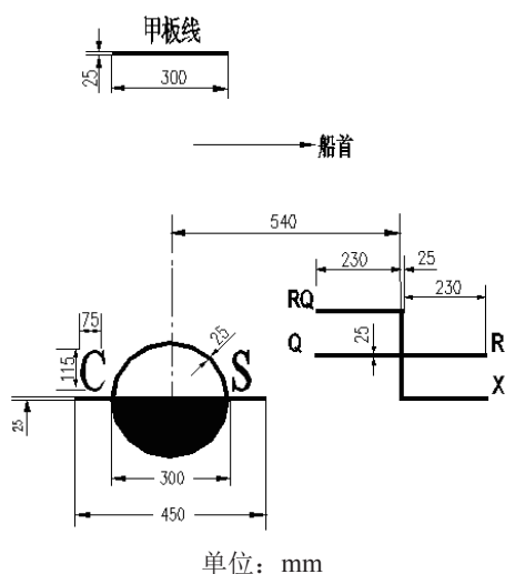
图2.1 不装载木材甲板货船舶的干舷标志
