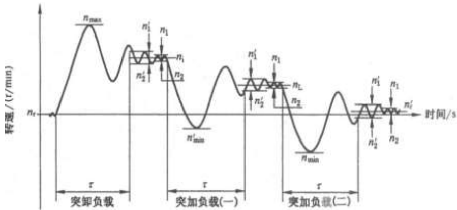
图 3.2(2) 转速调节
