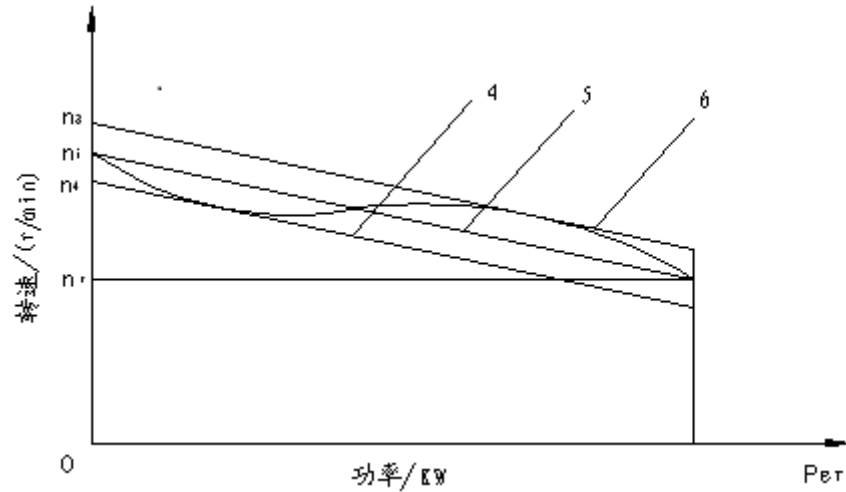
图 3.2(18) 调速特性的非直线度
