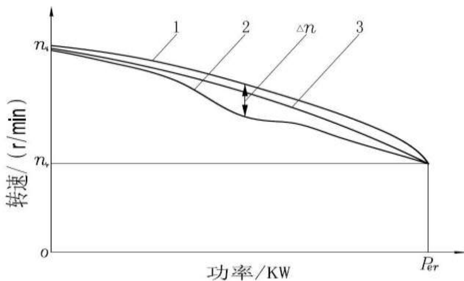
图 3.2(16) 调速特性曲线
