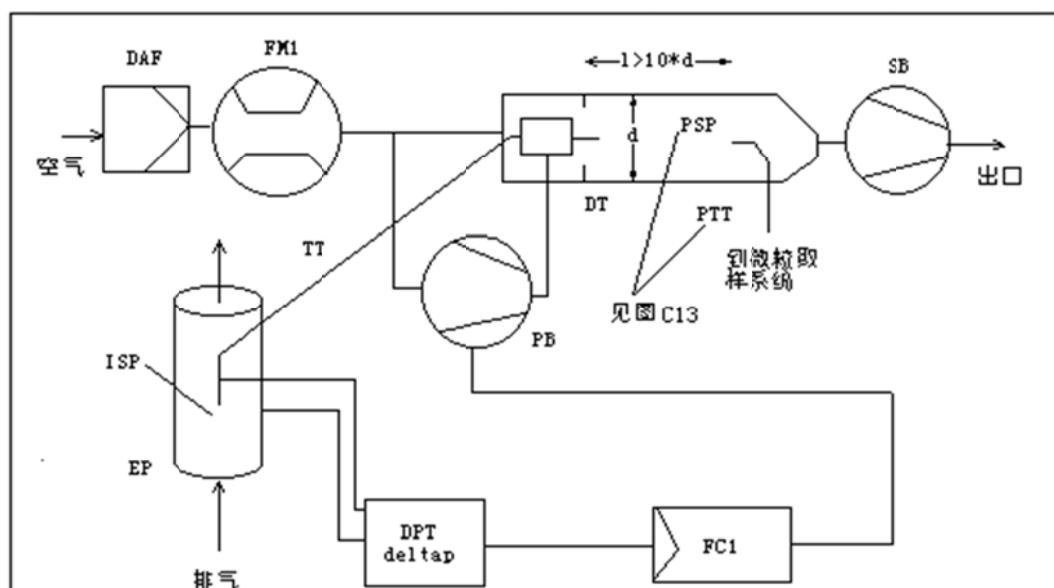
图 2.4 带等动态探头和部分流采样的部分流稀释系统(PB 控制)
