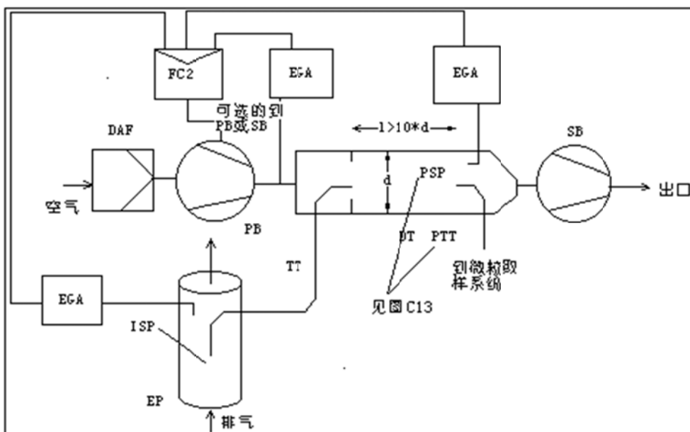
图 2.5 带 CO 2 和 NO x 浓度测量和部分流采样的部分流稀释系统
