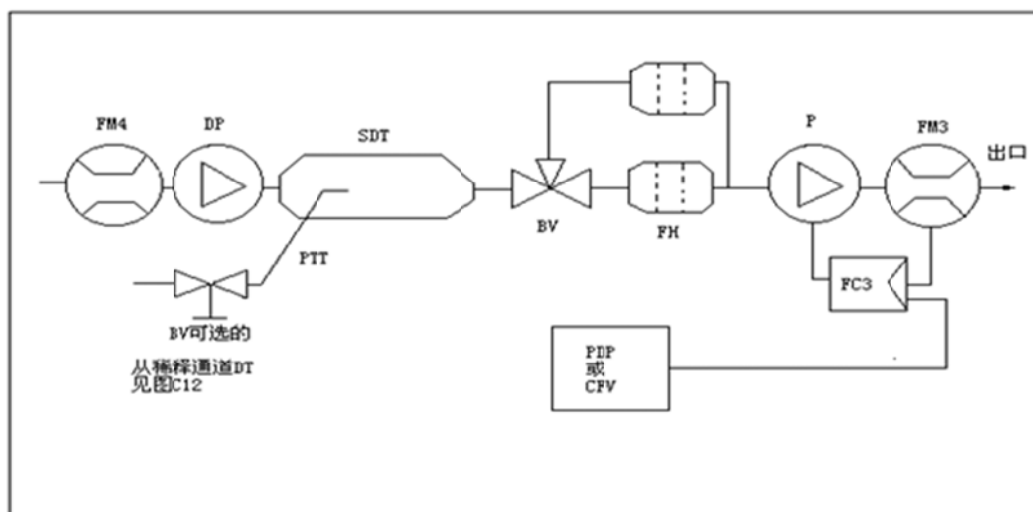
图 2.14 稀释系统(仅用于全流系统)
