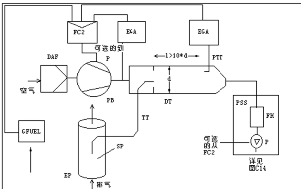
图 2.6 带 CO 2 浓度测量，碳平衡和全部取样的部分流稀释系统
