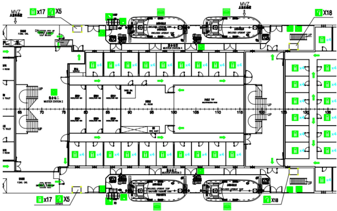
附图 2.1 某客船的救生艇布置局部图
