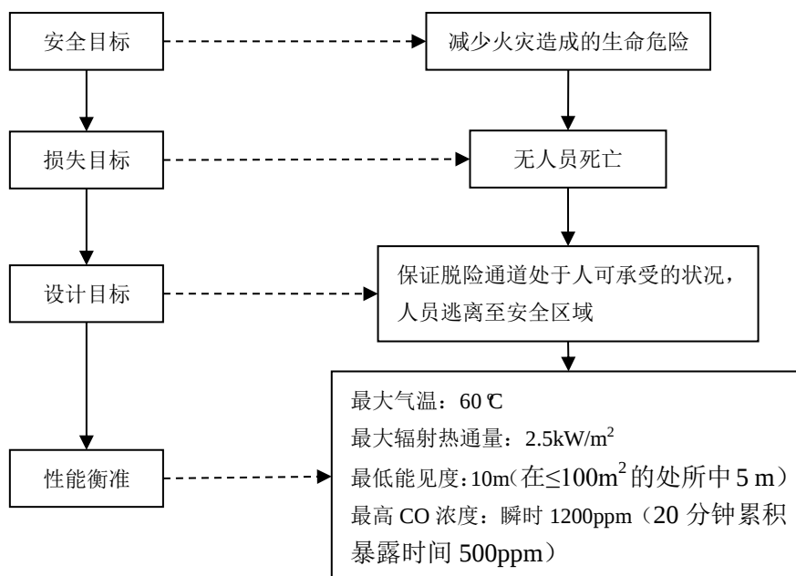
附图 1.1 人命安全性能衡准示例
