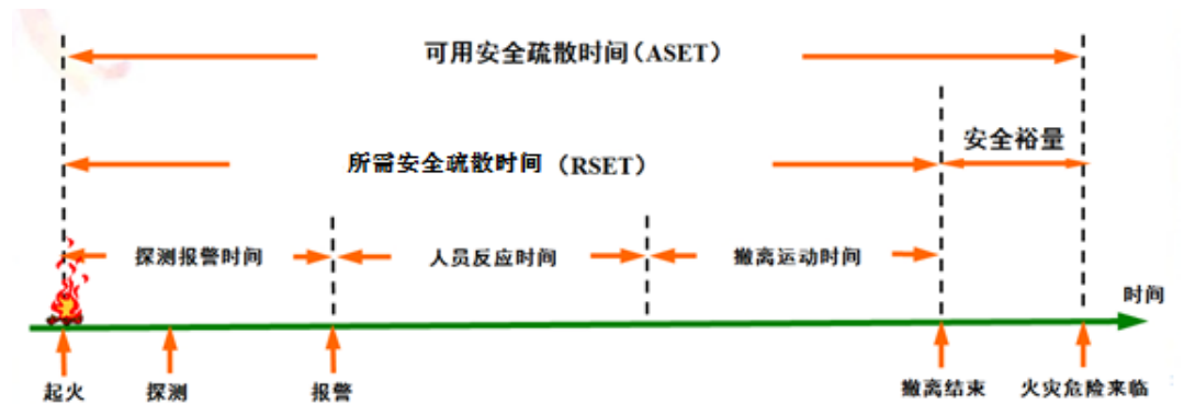
附图 1.2 人员撤离安全判定示意图
