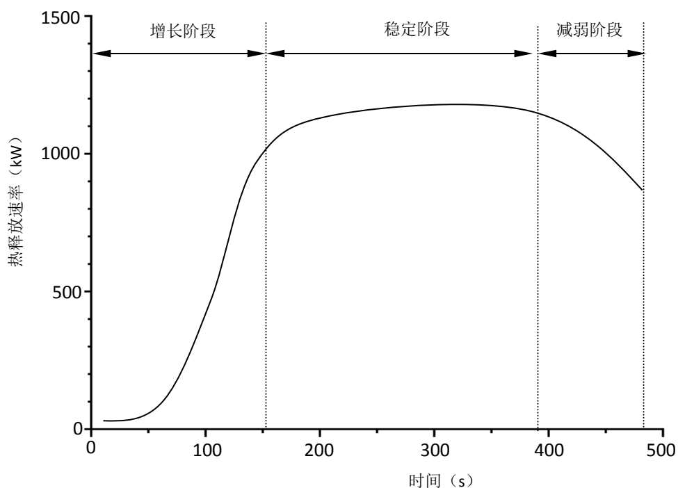
附图 1.4 火灾发展曲线示意图
