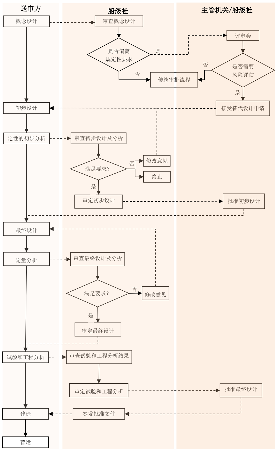
图 2.1 替代设计流程
