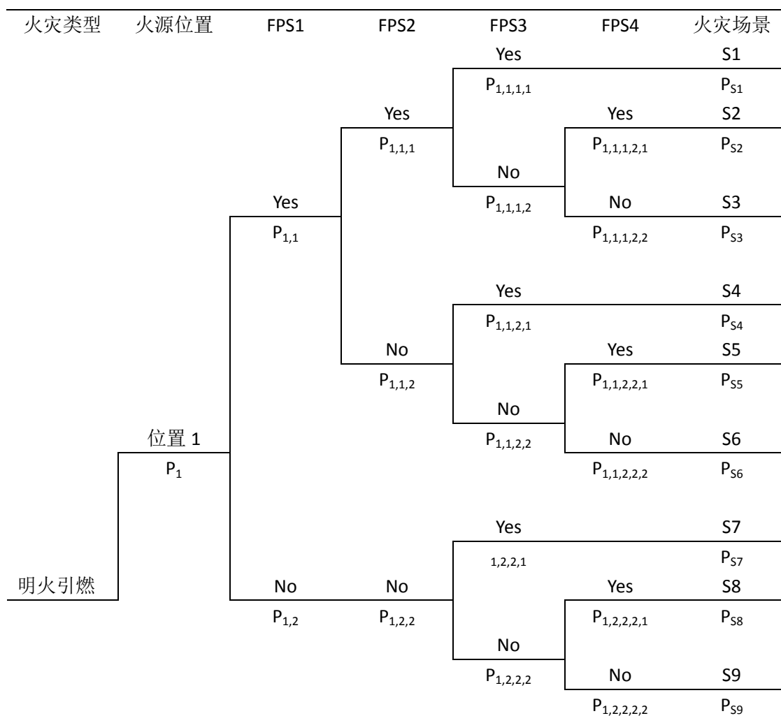
附图 1.3 火灾场景事件树示例图
