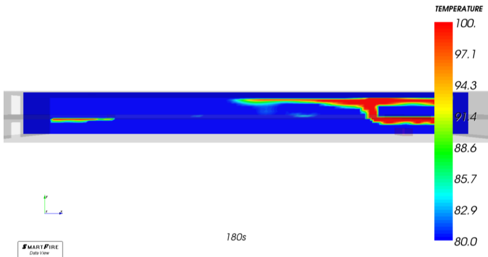
附图 1.9 火灾通过宴会厅下甲板和上甲板示意图
