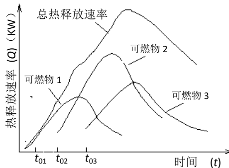
附图 1.5 可燃物依次着火总热释放速率的设定
