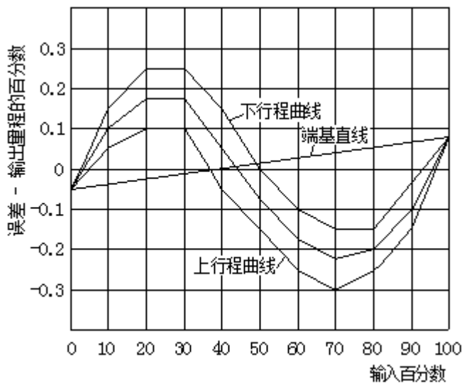
图 5.4.3(1) 偏差曲线
