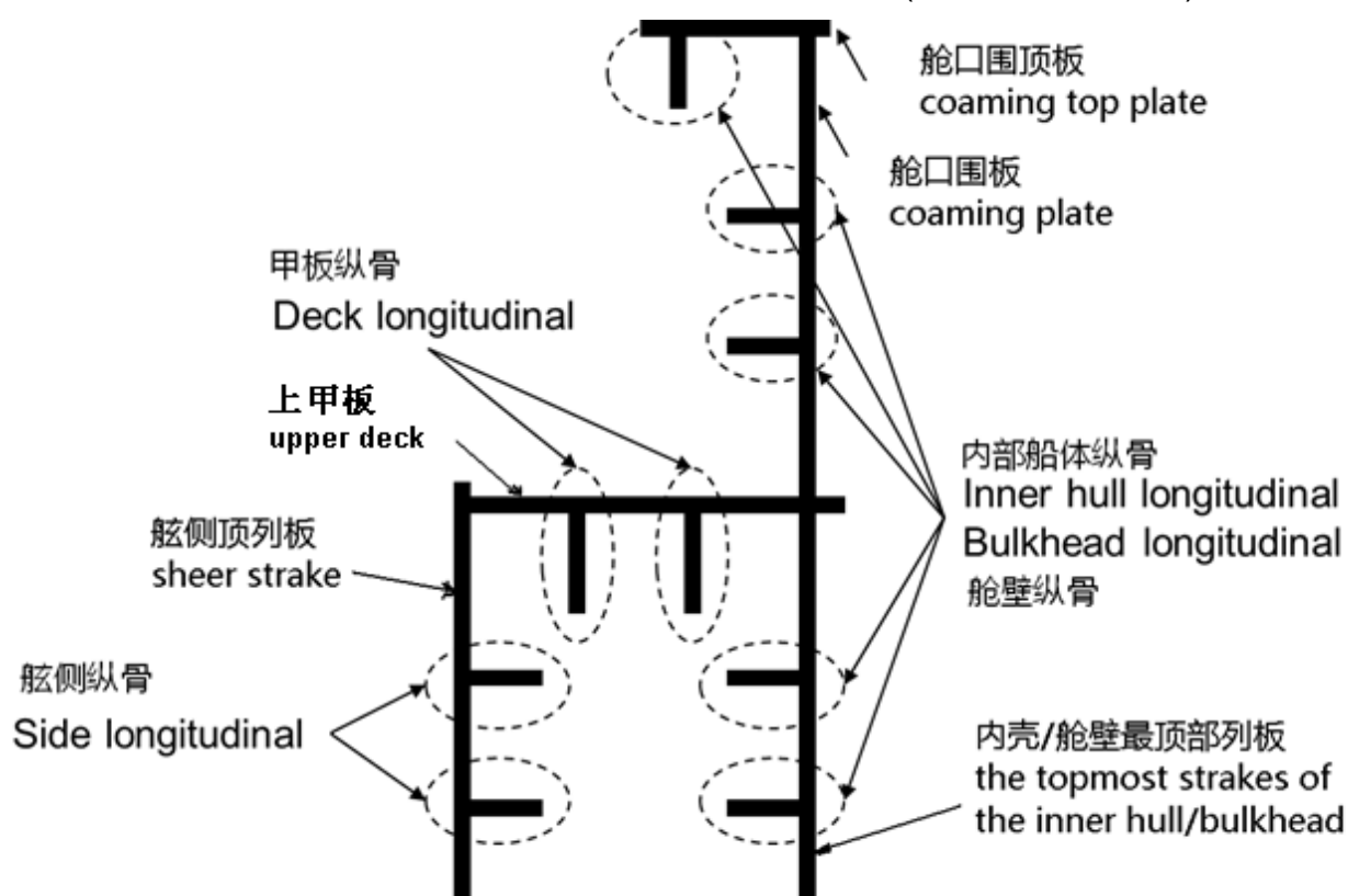
图 5.2.1 集装箱船货舱区域的纵向结构
