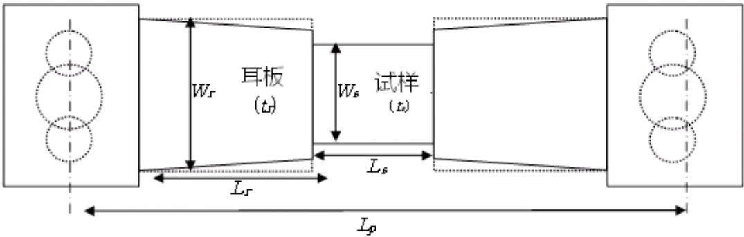
图 A 1 试样、连接板和加载夹具的概念
