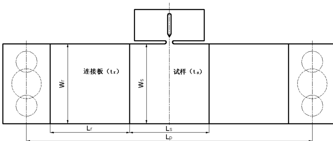
图B1 试样和连接板示意图
