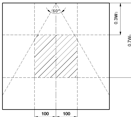
图 B3 裂纹有效止裂区域
