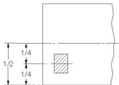
图 2.4.3 试件取样位置
