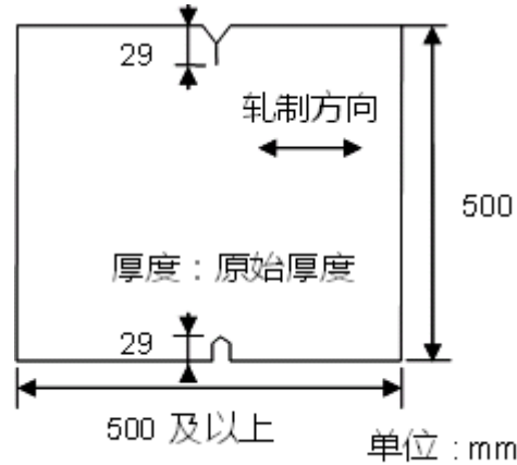
图 A 2 试样的形状和尺寸
