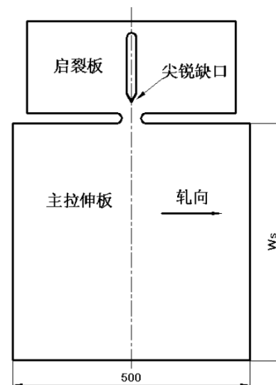
图B2 试样形式和尺寸
