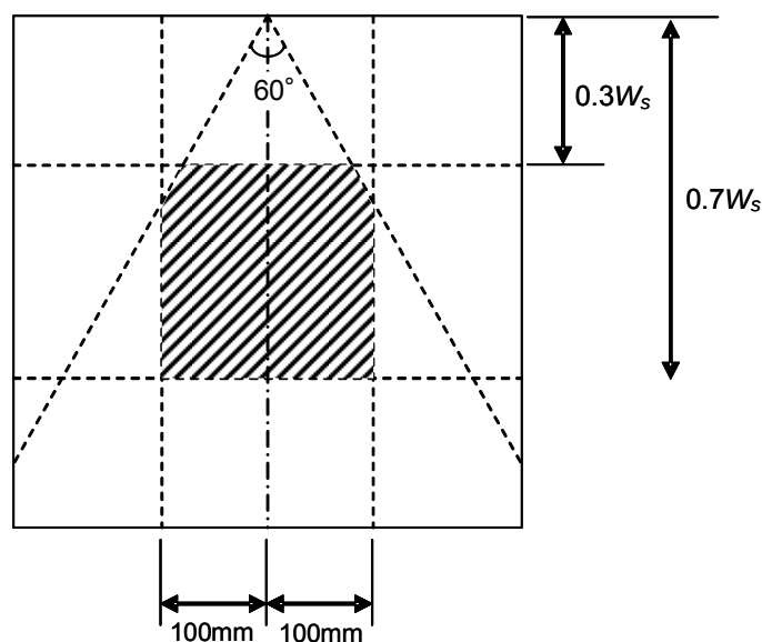
图 A 3 止裂位置的必要条件
