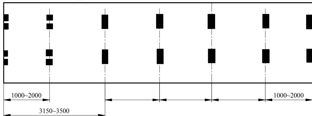
图 4.2.4.7(4) 带鹅颈槽的 1EEE、1EE、1AAA、1AA、1A 和 1AX 型集装箱的 7 对载荷传递区
