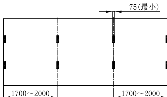
图 8.2.1.9 (1) 1C、1CC、1CX、1B、1BB、1BBB 和 1BX 型罐式集装箱的 2 对载荷传递区
