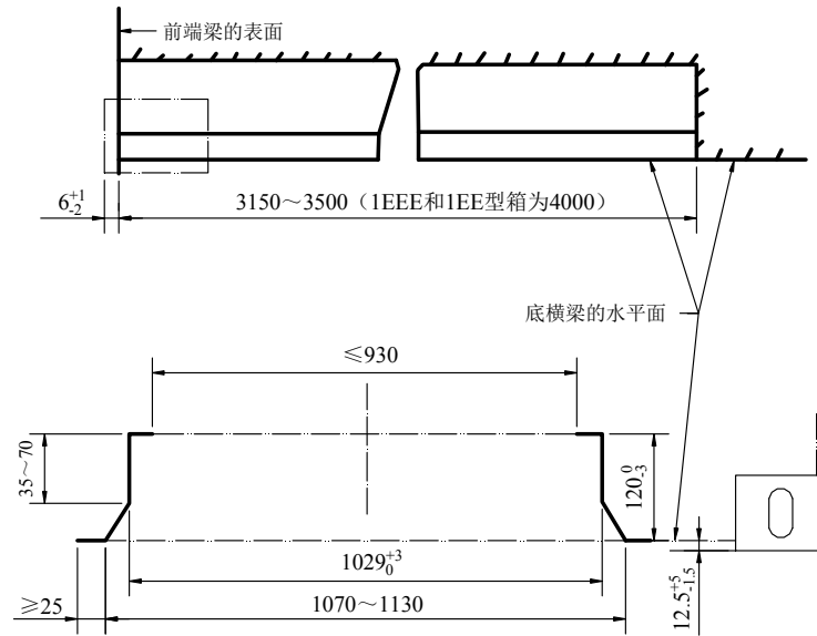
图 4.2.5.1(1) 鹅颈槽断面图 (单位: mm)
