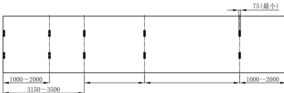
图 8.2.1.9 (3) 设鹅颈槽的 1A、1AA、1AAA 和 1AX 型罐式集装箱的 4 对载荷传递区
