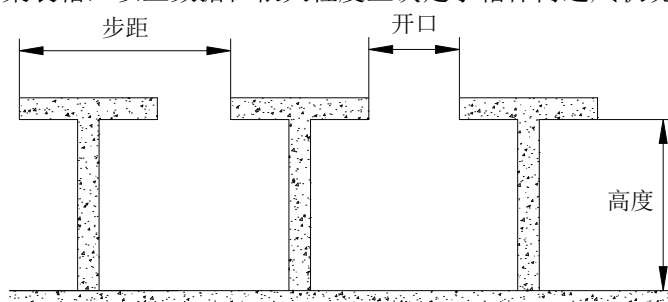
图 1.3 T-bars构造示意图
