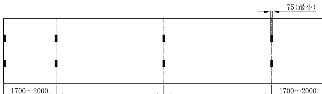
图 8.2.1.9 (2) 不设鹅颈槽的 1A、1AA、1AAA 和 1AX 型罐式集装箱的 3 对载荷传递区
