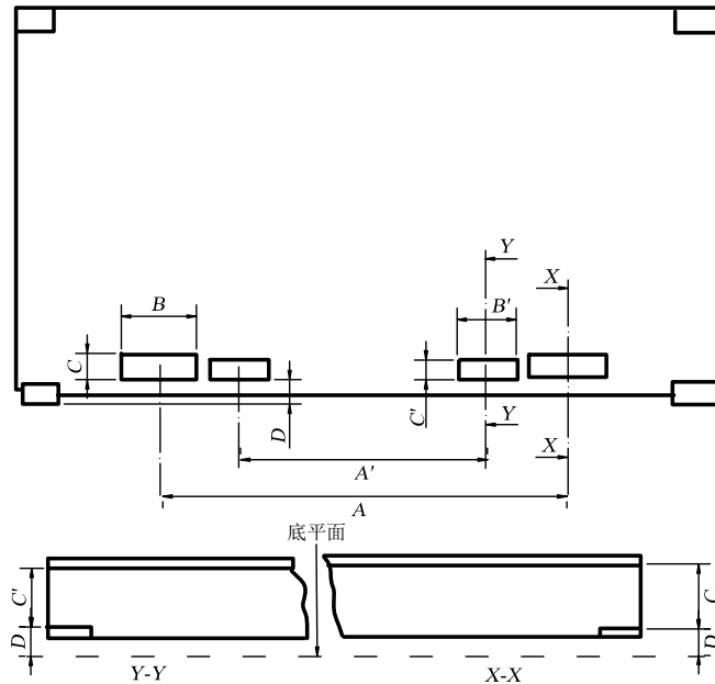
图 4.2.6.2 叉槽位置和尺寸示意图
