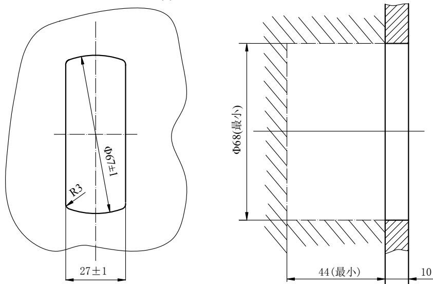
图 7.2.30(2) 放大详图
