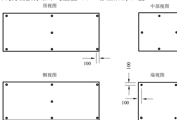
图 7.3.5.4(1) 箱内温度测点
