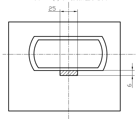
图 4.3.4(2) 底角件偏置时的承载面示意图 (单位: mm)
