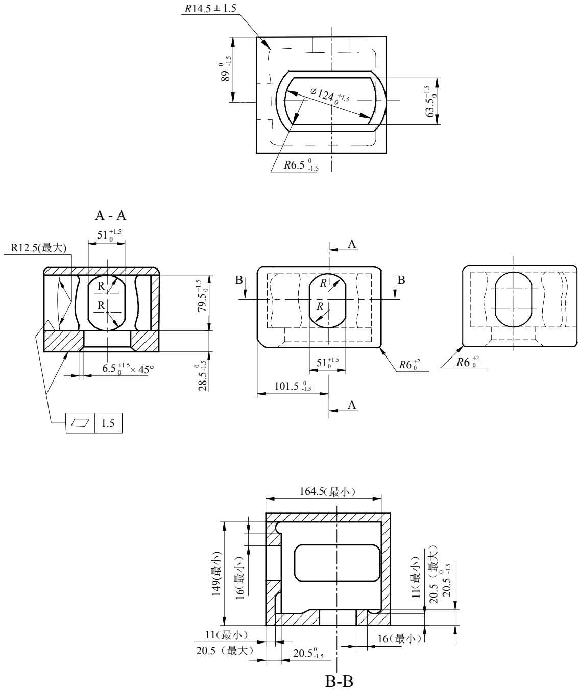
图 4.3.2(2) 底角件尺寸 (单位: mm)
