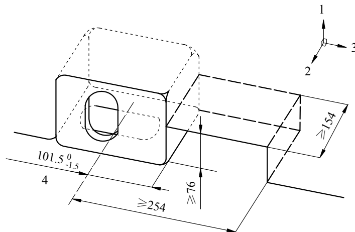
图 4.3.3 1EEE 和 1EE 型集装箱中间底角件的凹槽（单位：mm）
