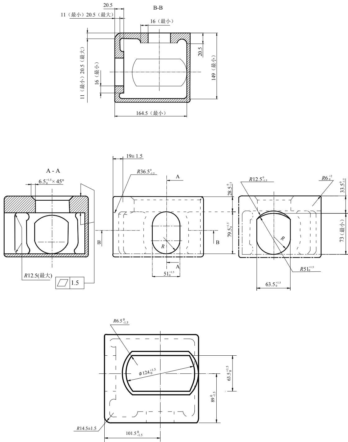
图 4.3.2(1) 顶角件尺寸 (单位: mm)
