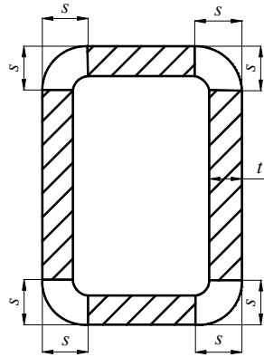
图 3.3.4.1 方形钢管尺寸示意图
