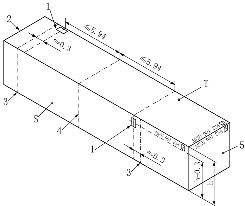
图 10.8.2.2 (1) 箱长小于或等于 12.2m 时标签安装位置示意图
