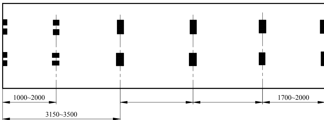
图 4.2.4.6(4) 带鹅颈槽的 1AAA、1AA、1A 和 1AX 型集装箱的 6 对载荷传递区
