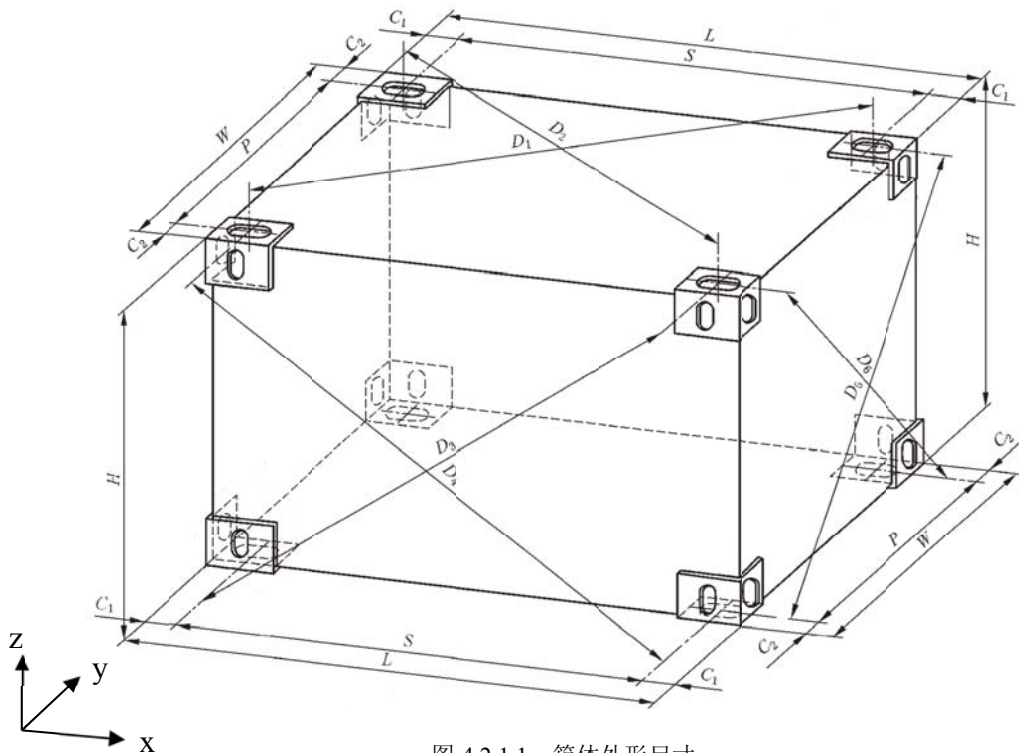
图 4.2.1.1 箱体外形尺寸
