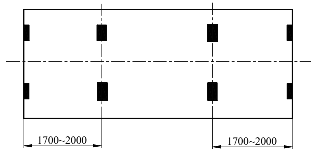
图 4.2.4.6(1) ICC、1C 和 1CX 型集装箱的 4 对载荷传递区
