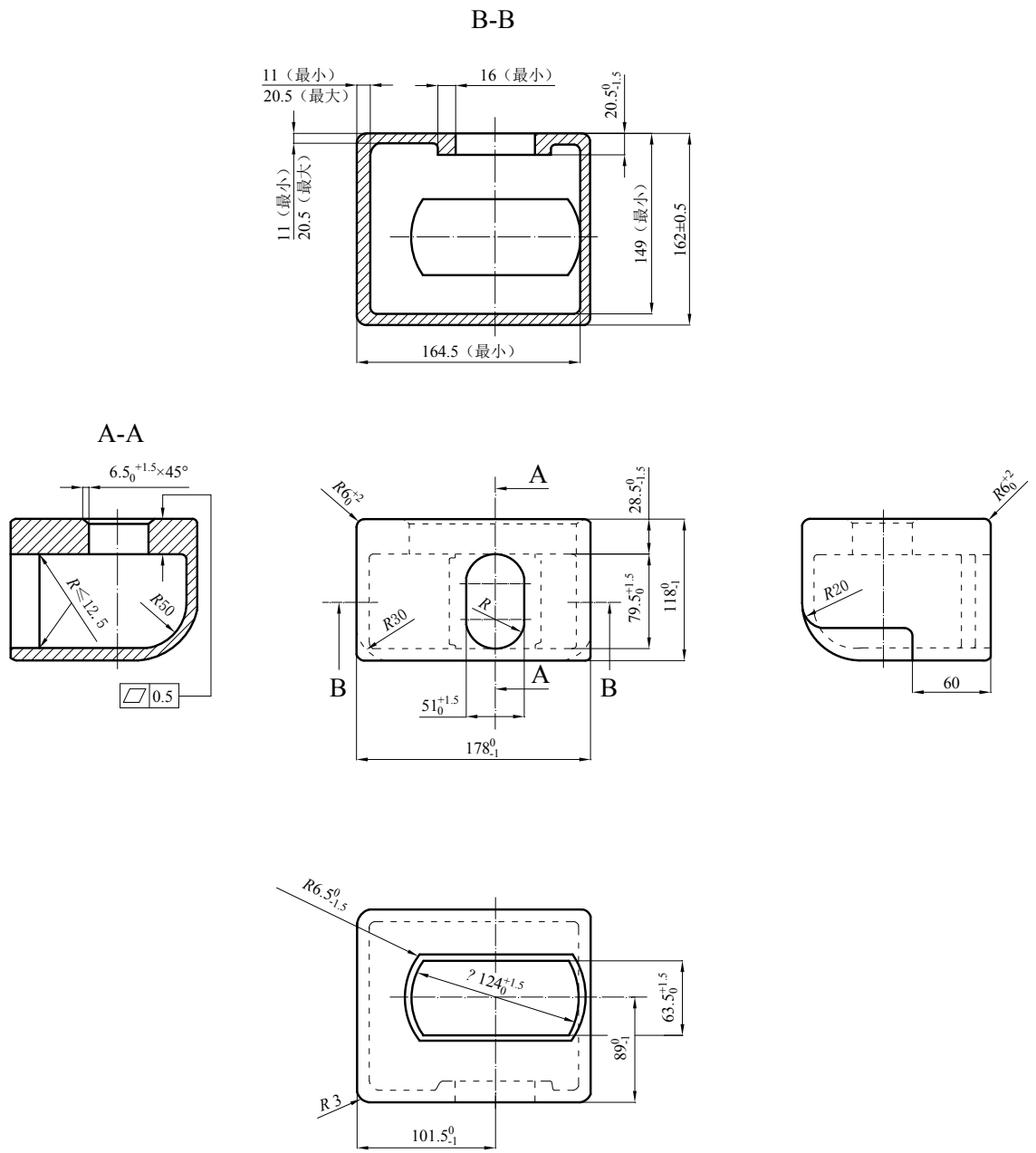
图 4.3.2(3) 中间顶角件尺寸 (单位: mm)
