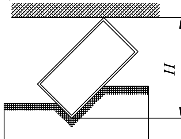
图 3.3.7.2 方管压扁试验示意图
