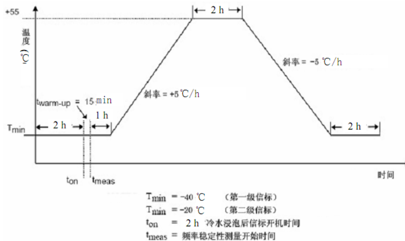
图 5.2.18 温度梯度
