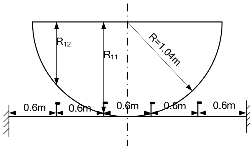
附图 7 球形撞头撞击外壳板示意图
