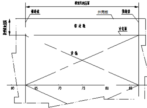
图 3.3.5.1 被撞船有限元模型范围示意图
