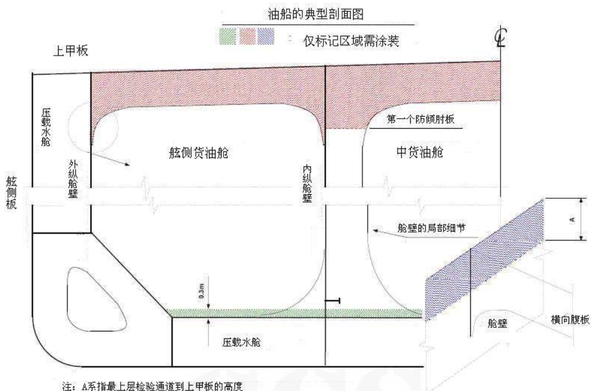
图 5.3.2 原油船货油舱的涂装区域
