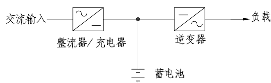
图 1.1.2.1 (30) 在线式 UPS 装置示意图
