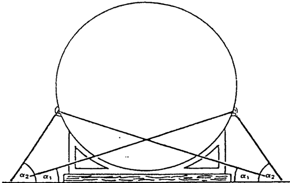
图 1 以有利的绑绳角度系固移动式罐柜
